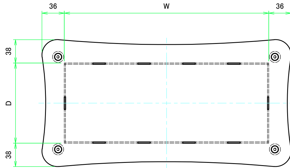
上カバー / Top cover
