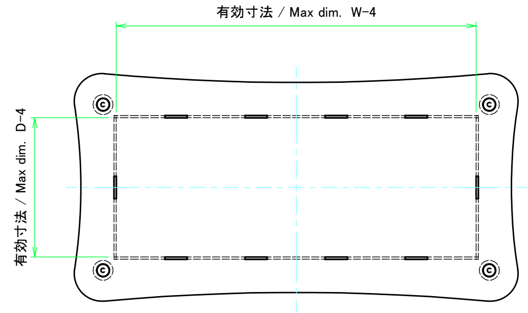
下カバー / Bottom cover
