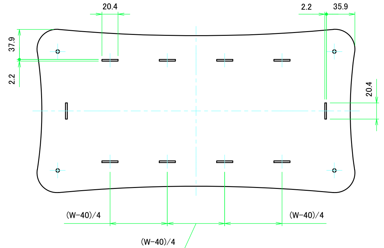
上カバー裏面 / Top cover Backside
