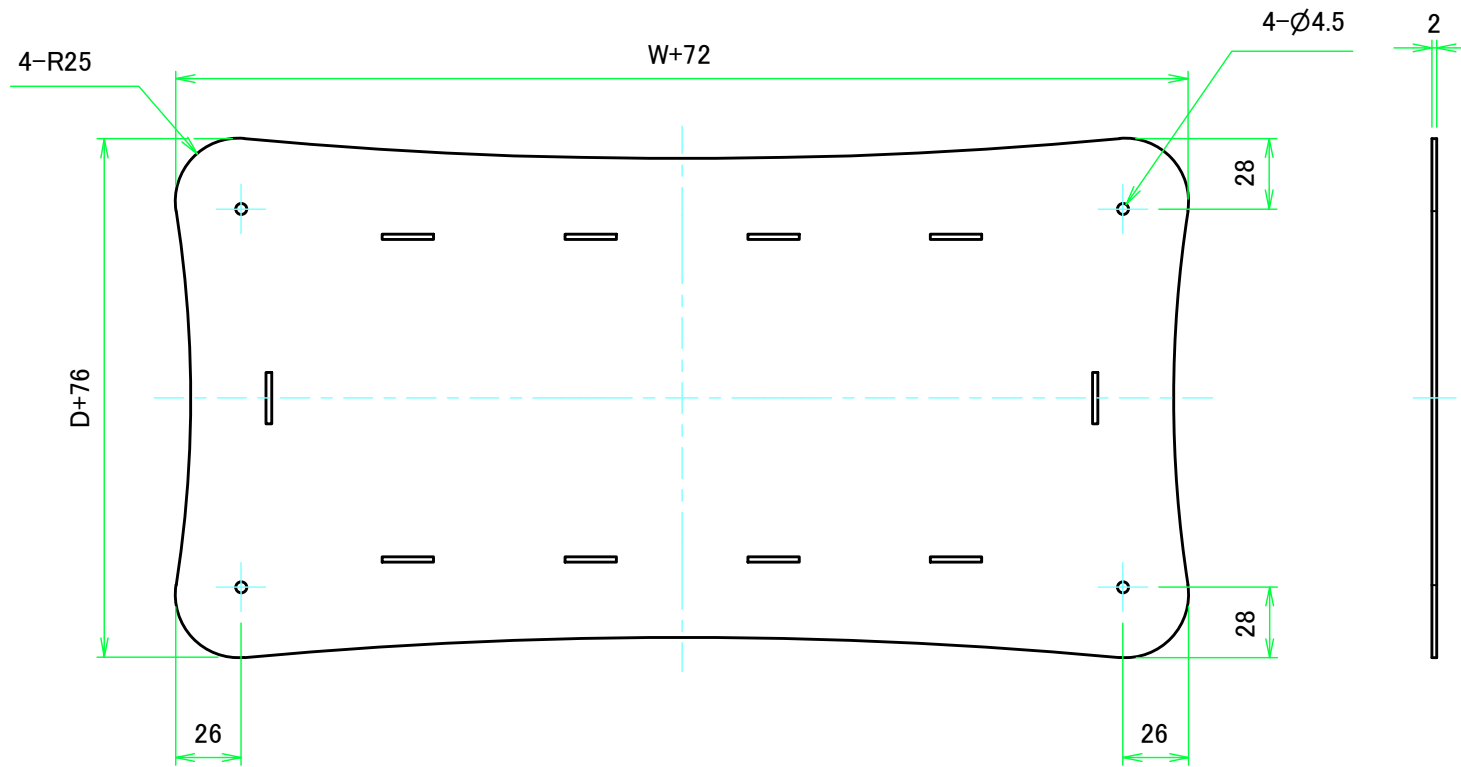
上カバー表面 / Top cover Frontside
